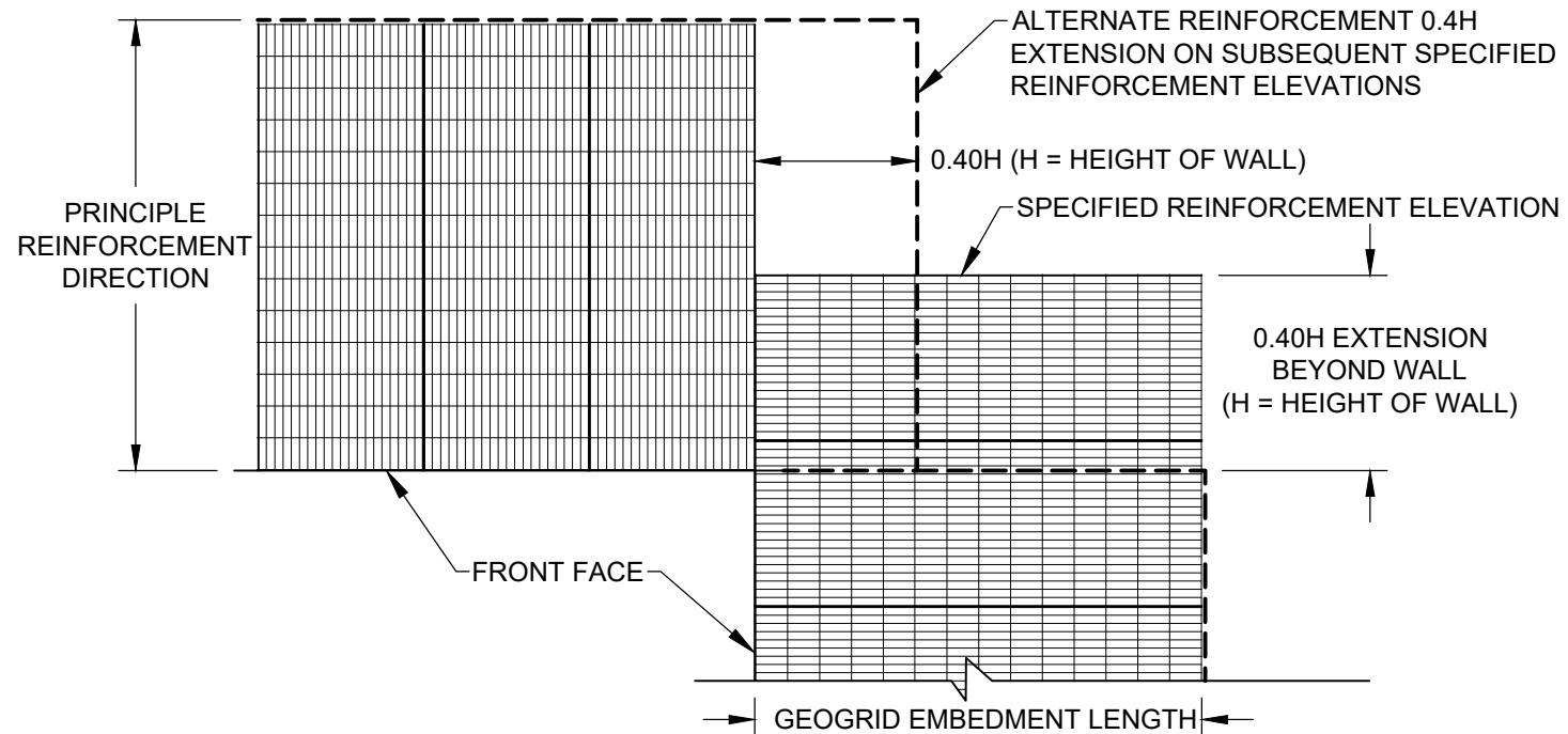
INSIDE CORNER REINFORCEMENT LAYOUT DETAIL (N.T.S.)
